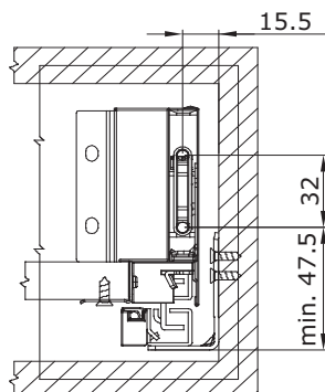
Wymiary montażowe frontu /Front panel installation dimensions
