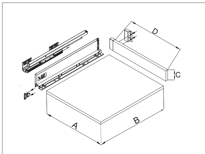
Wymiary wewnętrzne korpusu /Internal cabinet dimensions
