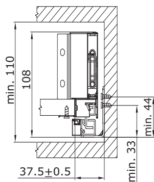
Wymiary wewnętrzne korpusu /Internal cabinet dimensions
