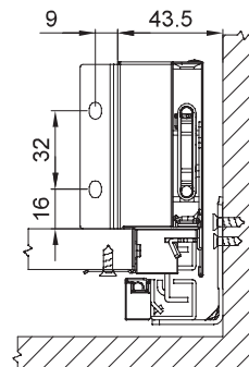
Wymiary montażowe panelu tylnego / Back panel installation dimensions
