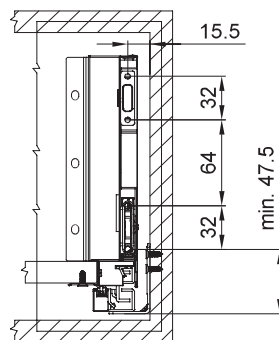
Wymiary montażowe frontu / Front panel installation dimensions
