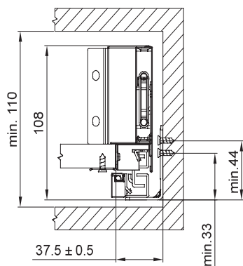
Wymiary wewnętrzne korpusu / Internal cabinet dimensions
