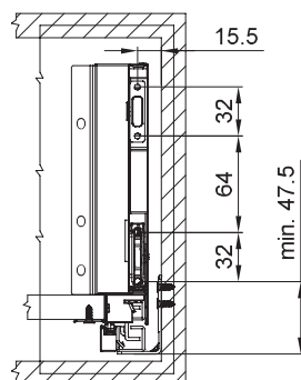
Wymiary montażowe frontu / Front panel installation dimensions
