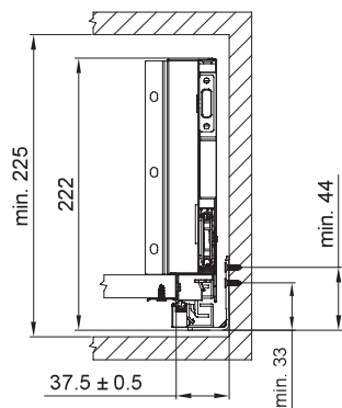
Wymiary wewnętrzne korpusu / Internal cabinet dimensions
