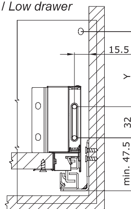
Szuflada niska / Low drawer
