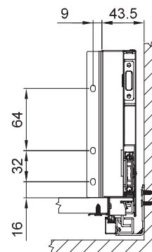
Wymiary montażowe panelu tylnego / Back panel installation dimensions
