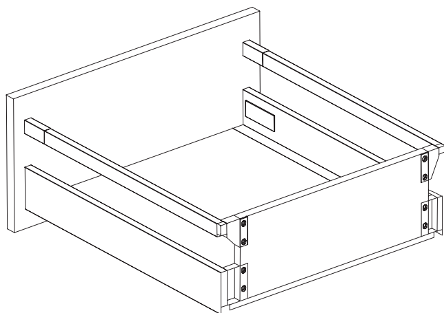
Szuflada średnia / Medium drawer
