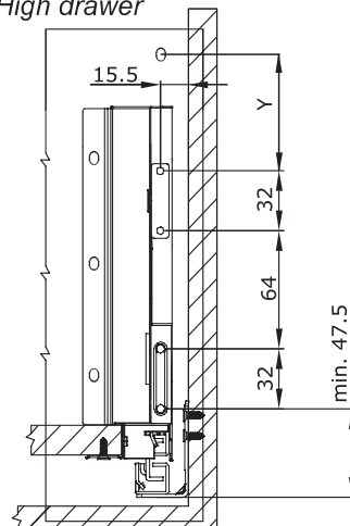
Szuflada wysoka / High drawer
