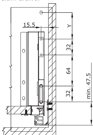
Szuflada średnia / Medium drawer
