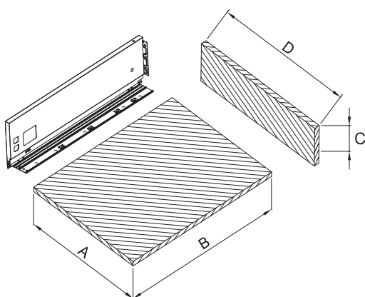
Wymiary wewnętrzne korpusu / Internal cabinet dimensions
