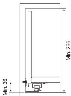
Wymiary wewnętrzne korpusu / Internal cabinet dimensions
