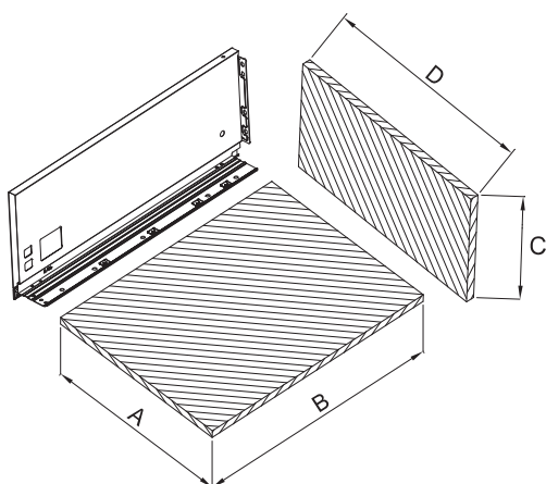
Wymiary wewnętrzne korpusu / Internal cabinet dimensions
