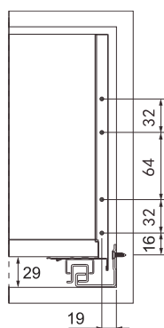
Wymiary montażowe frontu / Front panel installation dimensions
