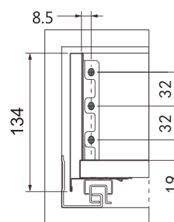
Wymiary montażowe panelu tylnego / Back panel installation dimensions
