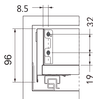
Wymiary montażowe panelu tylnego / Back panel installation dimensions
